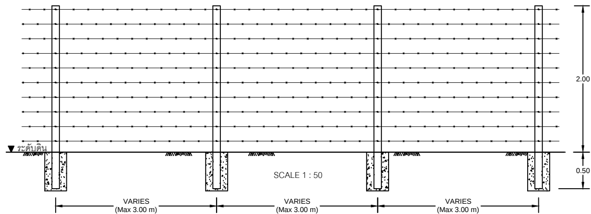
แบบการติดตั้งรั้วลวดหนาม 2.5 m. 4" x 4" scale 1:50
