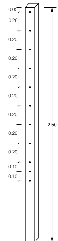
แบบขยายเสา
