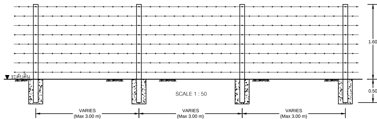
แบบการติดตั้งรั้วลวดหนาม 2.1 m. 4" x 4" scale 1:50
