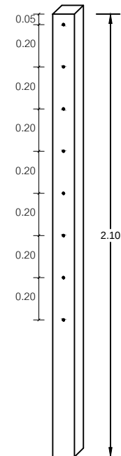
แบบขยายเสา
